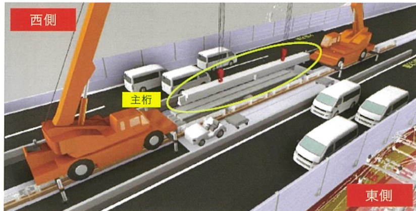
幅員減少規制①橋の架け替えイメージ
