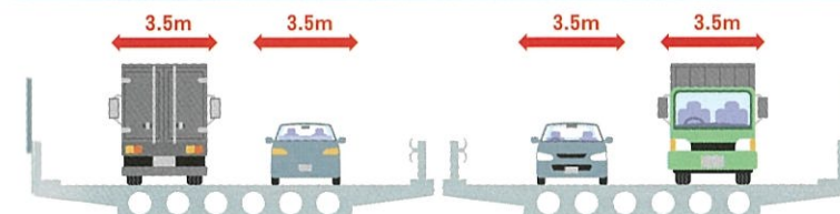
現況 断面図
